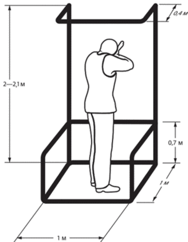
Рисунок 2-1. Устройство стрелкового места для "спортинг-компакта".
